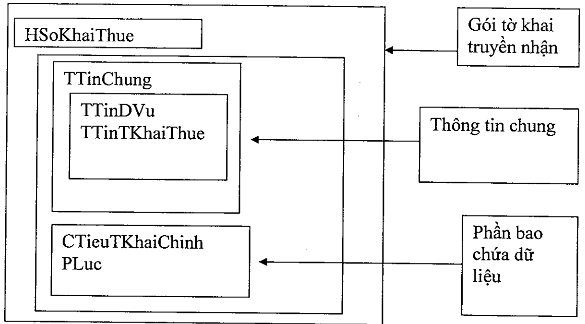
Hình minh họa 1: Định dạng của một tờ khai được mô tả dưới dạng hình khối
