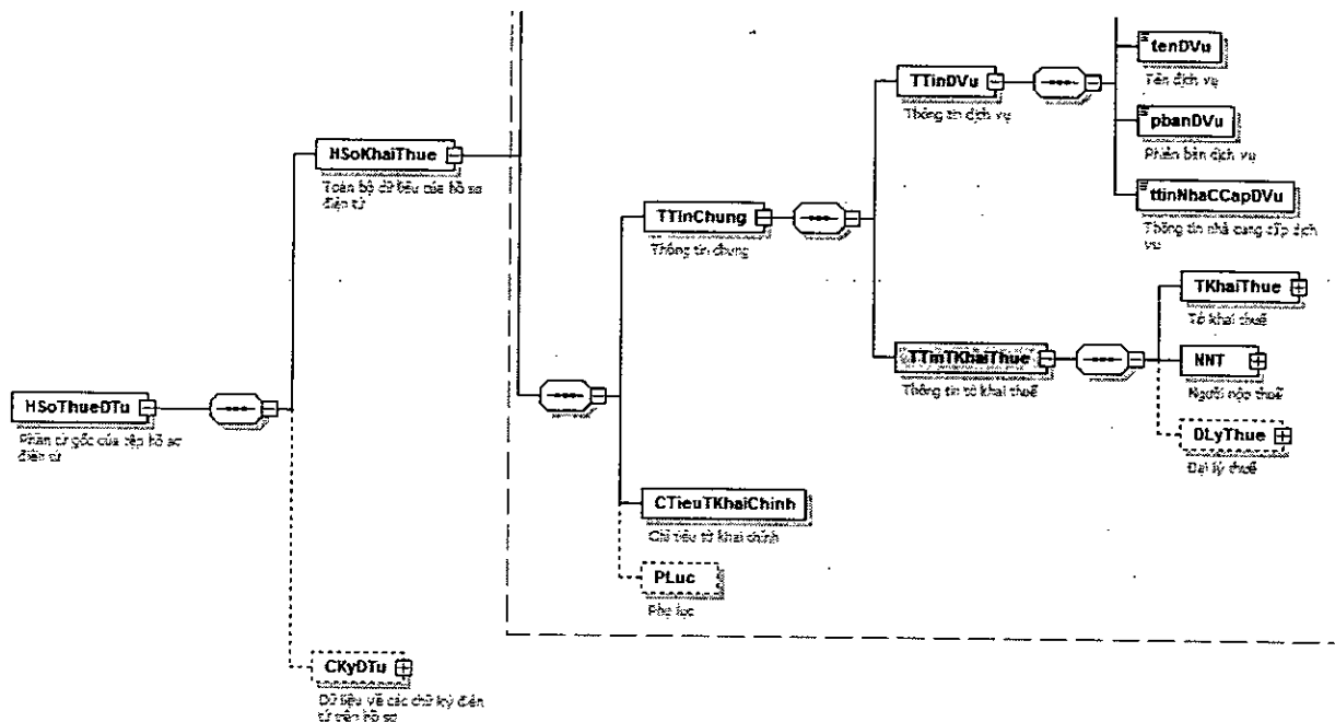
Hình minh họa 2: Định dạng của một tờ khai được mô tả dưới dạng hình cây
